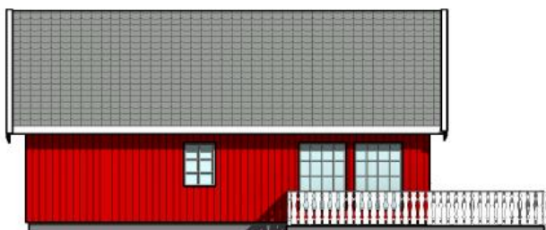
Fasade mot VEST 1 : 100
