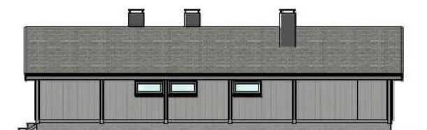
Fasade øst
